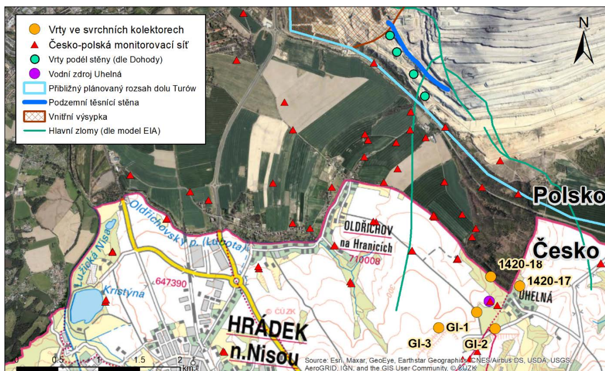
Obr. 6: Umístění vrtů ve svrchním kolektoru v okolí Uhelné
