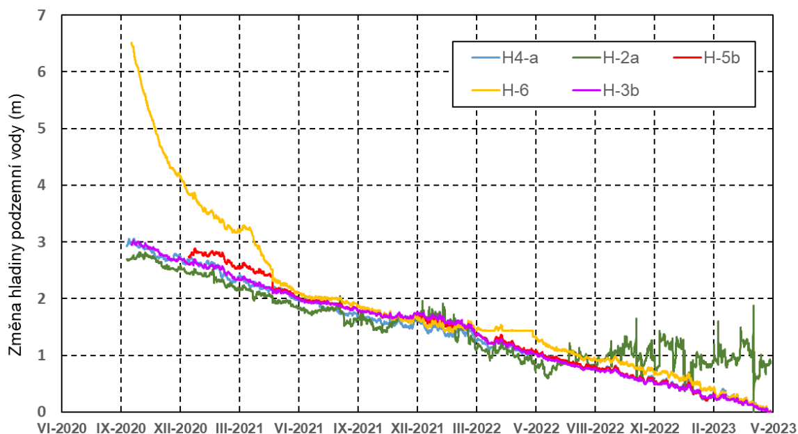
Obr. 3: Vývoj hladiny podzemní vody v hlubších kolektorech na českém území
