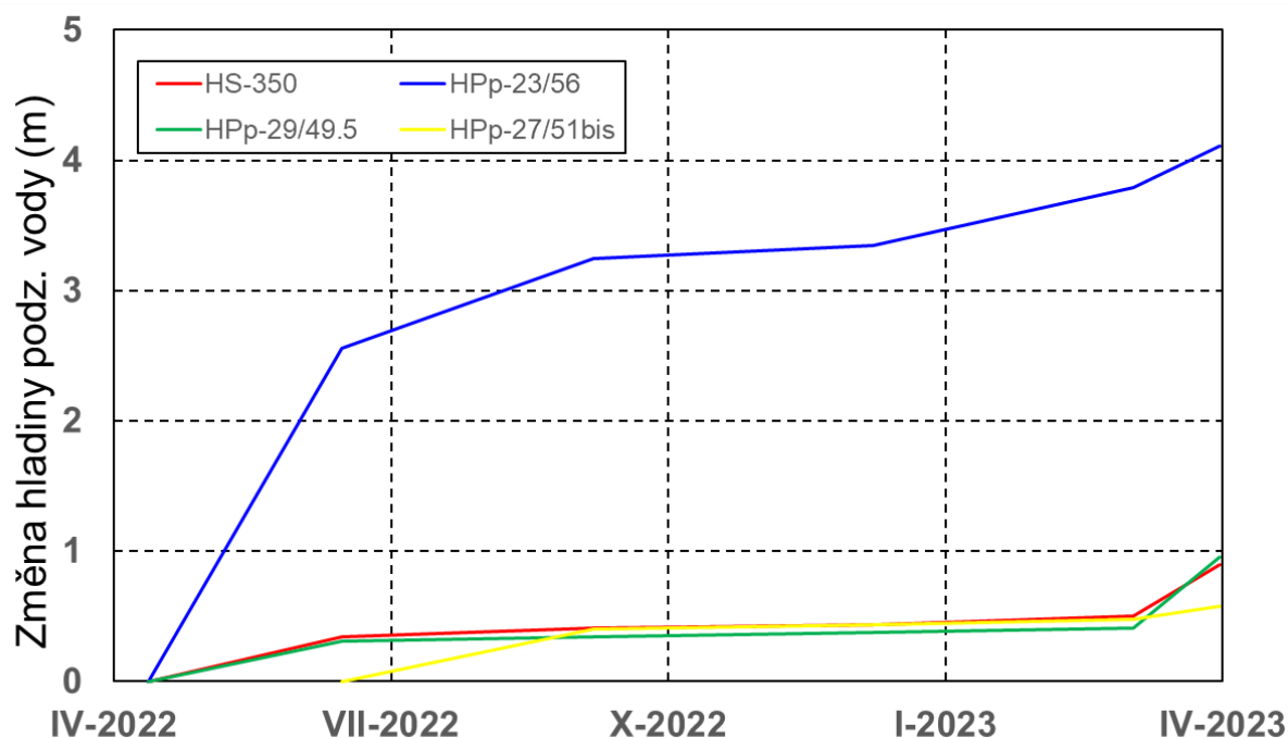
Obr. 1: Vývoj změny hladin na vrtech uvedených v Dohodě k posuzování k funkčnosti podzemní těsnicí stěny
