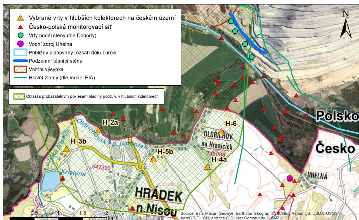
Obr. 4: Umístění vybraných vrtů v hlubších kolektorech na českém území
