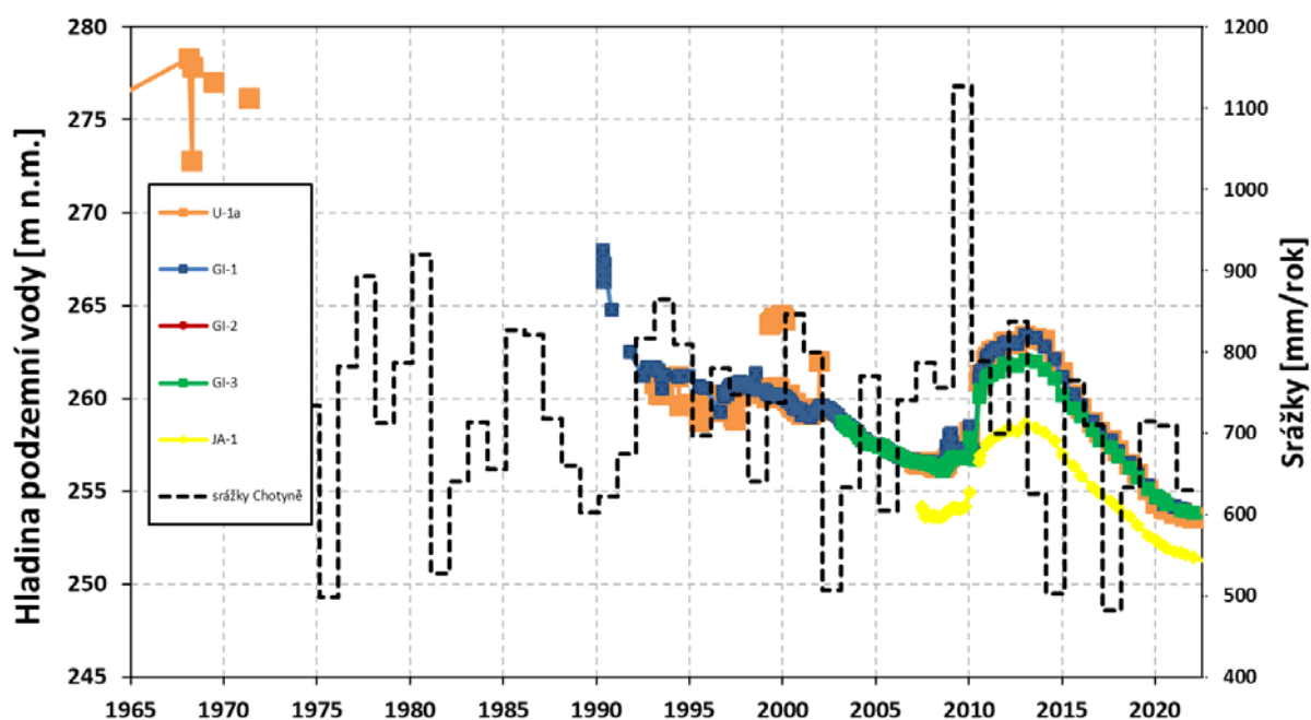
Obr. 7: Dlouhodobý vývoj hladiny podzemní vody ve svrchních kolektorech v okolí Uhelné
