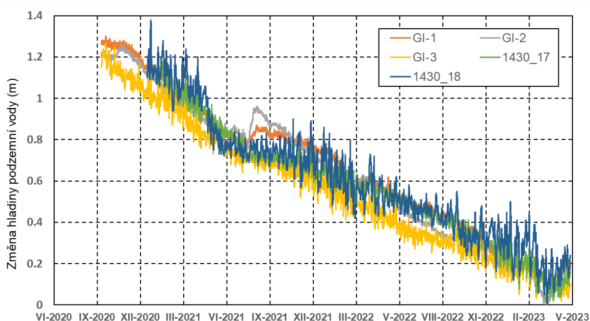
Obr. 5: Vývoj hladiny podzemní vody ve svrchních kolektorech v okolí Uhelné
