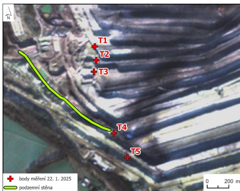
Obr. 2. Situace míst s realizovanými hydrologickými měřeními 22.1.2025 na snímku družice Sentinel.
