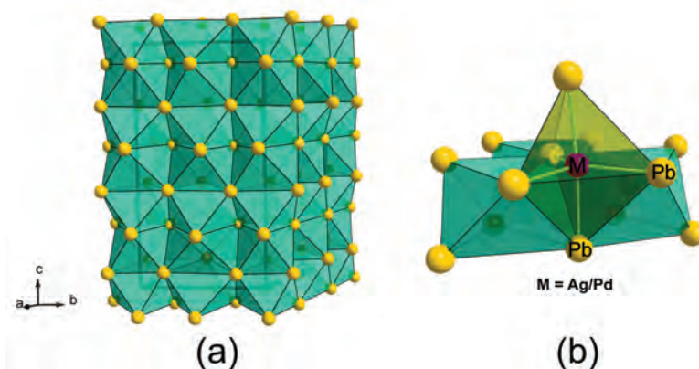
Krystalová struktura nového minerálu norilskitu, (\text{Ag,Pd})_{7-x}\text{Pb}_4 , (a) struktura znázorněná pomocí koordinačních polyedrů [\text{MPb}_6] , (b) detailní pohled znázorňující obsazení pozic v jedné vrstvě.
