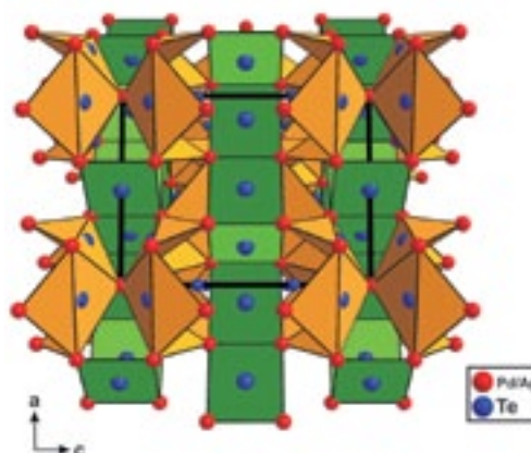
■ Krytalová struktura nového minerálu lukkulaivaaraitu, Pd 14 Ag 2 Te 9 .
